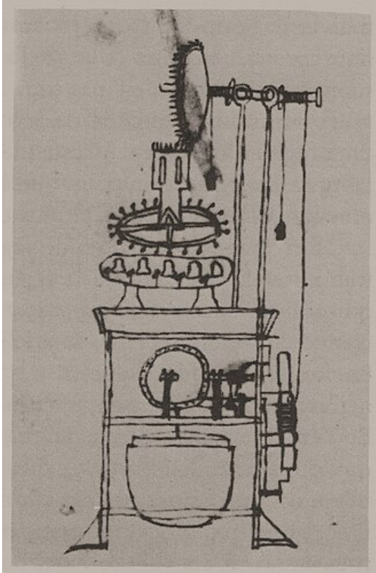
Horloge hydrolique
